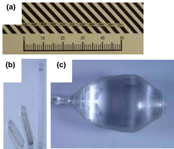
図1 \mu -PD法及びCz法で作製した Ce:Gd 0.5 Y 0.5 F 3 単結晶(a), Pr:LuAG単結晶(b),(c)
