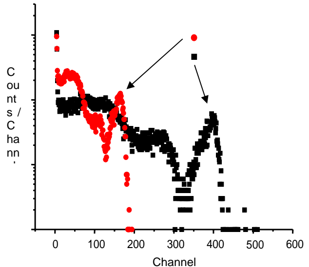
図2 Pr:LuAG単結晶のBGOとの発光量の比較
